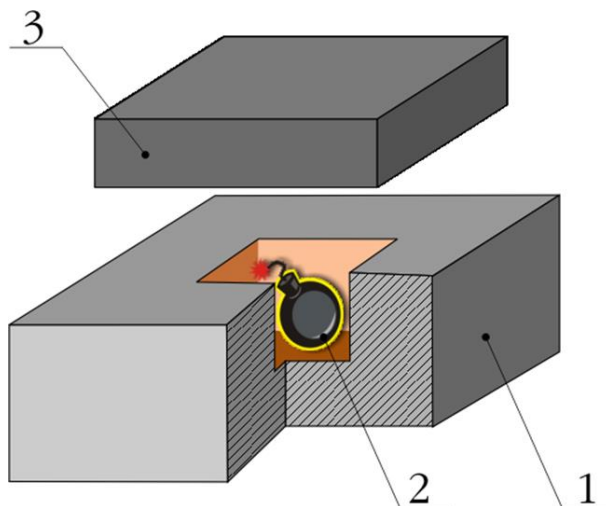
1 – Корпус устройства для защиты от взрыва 2 – Внутренняя полость для размещения взрывоопасного предмета 3 – Крышка
